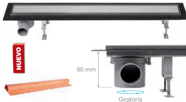
Canaleta Brillance 800 mm con válvula 75 mm · Fabricada en acero inoxidable AISI 304 · Válvula de 75 mm con salida a desagüe de Ø 50 mm
