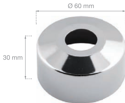
Florón doble bombeado \varnothing 1/2" \text{ G.}
