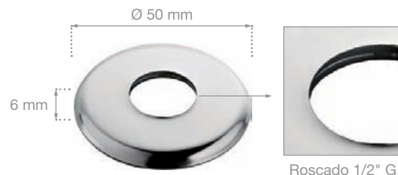
Florón inox bombeado con rosca 1/2'' \text{ G.}
